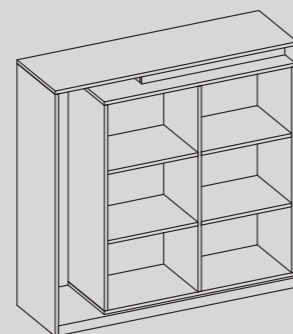
AN-38 126,8/ 40/H126,8
