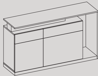
AN-21 146,8/40/H83,5
